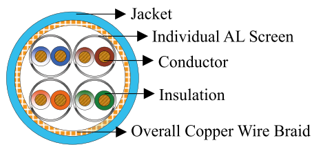
Cat6A S/FTP
