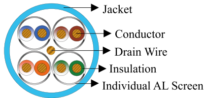
Cat6A U/FTP
